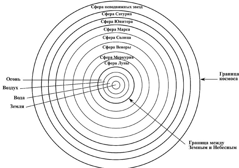
Система гомоцентрических сфер Аристотеля
