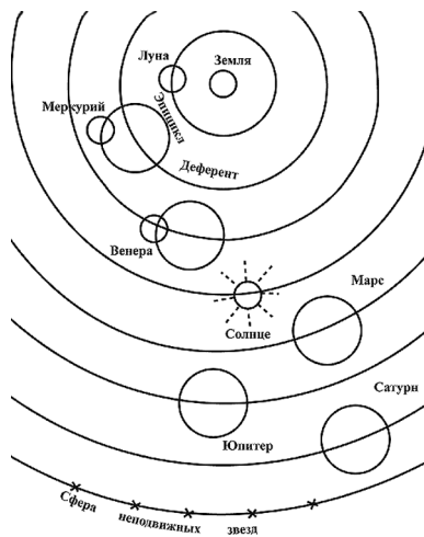
Система сфер согласно Маймониду
